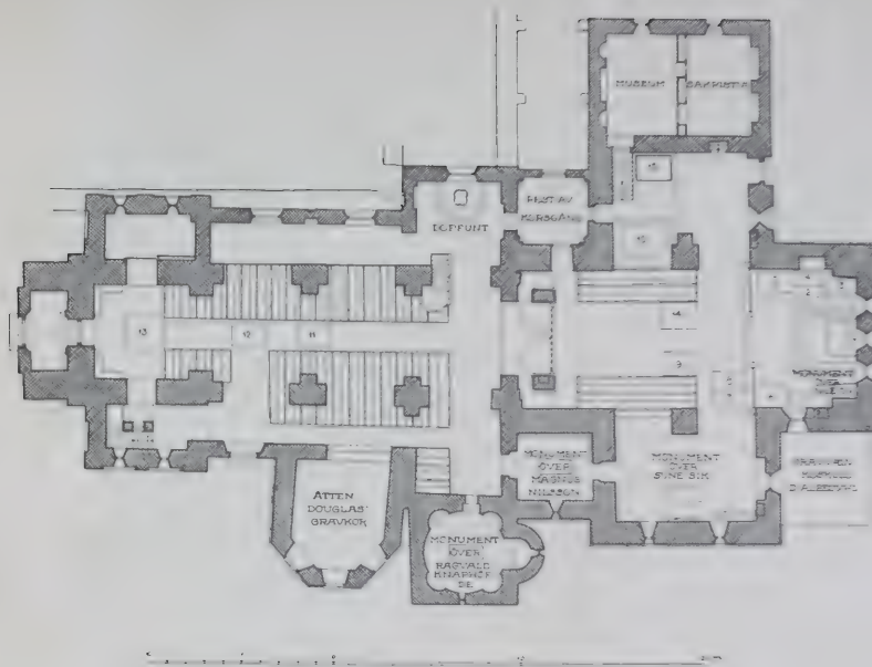
Plan av kyrkan 1917.
